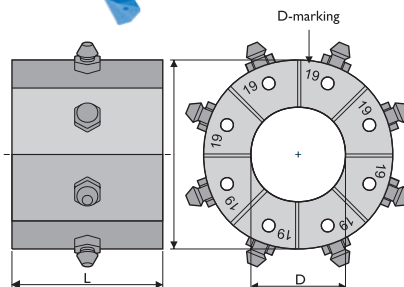
Tool base (part no 719124)
